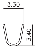
A-A SEC
